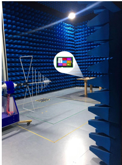
图 4-4 RE 测试图
